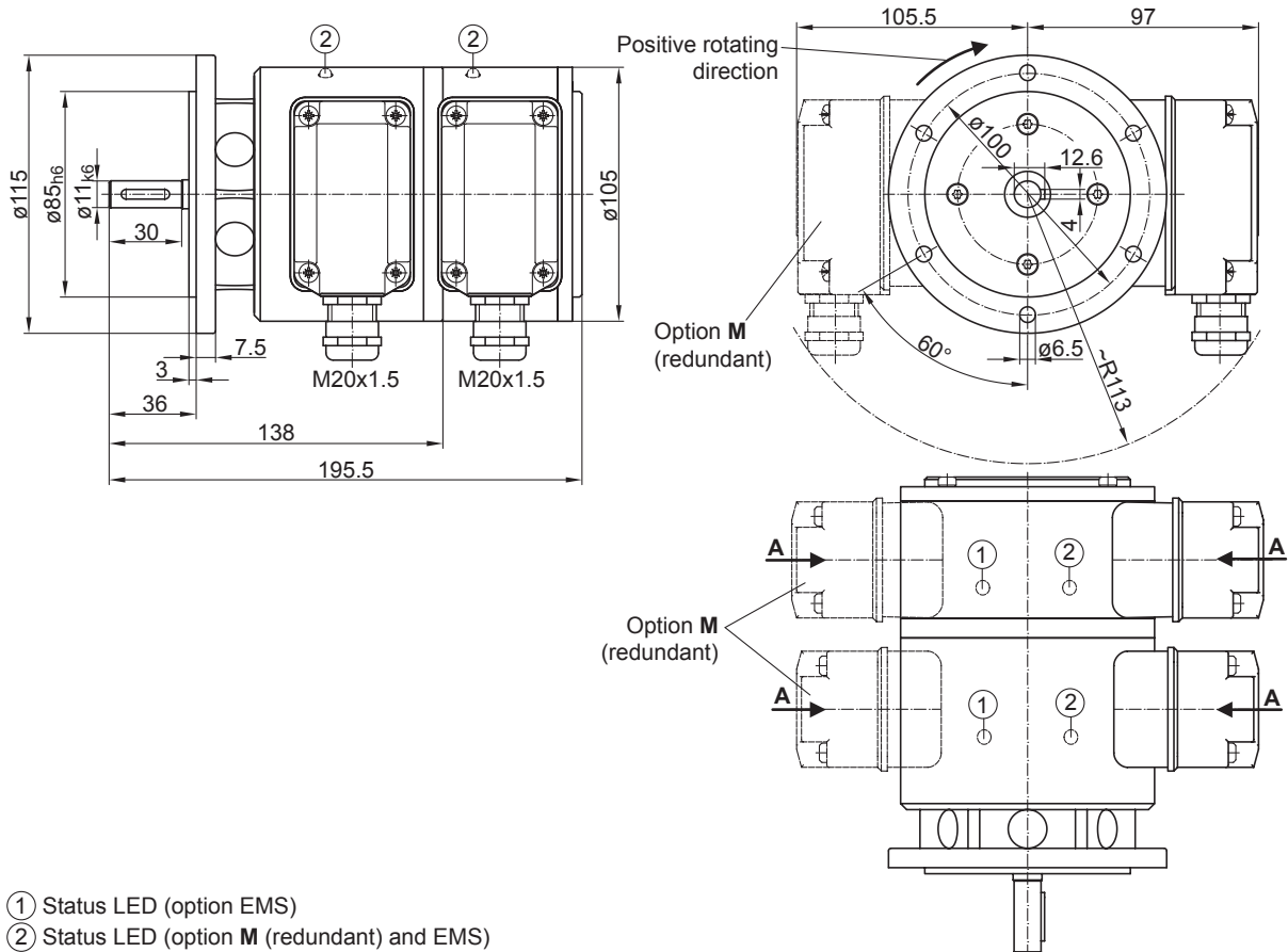
EURO flange B10
